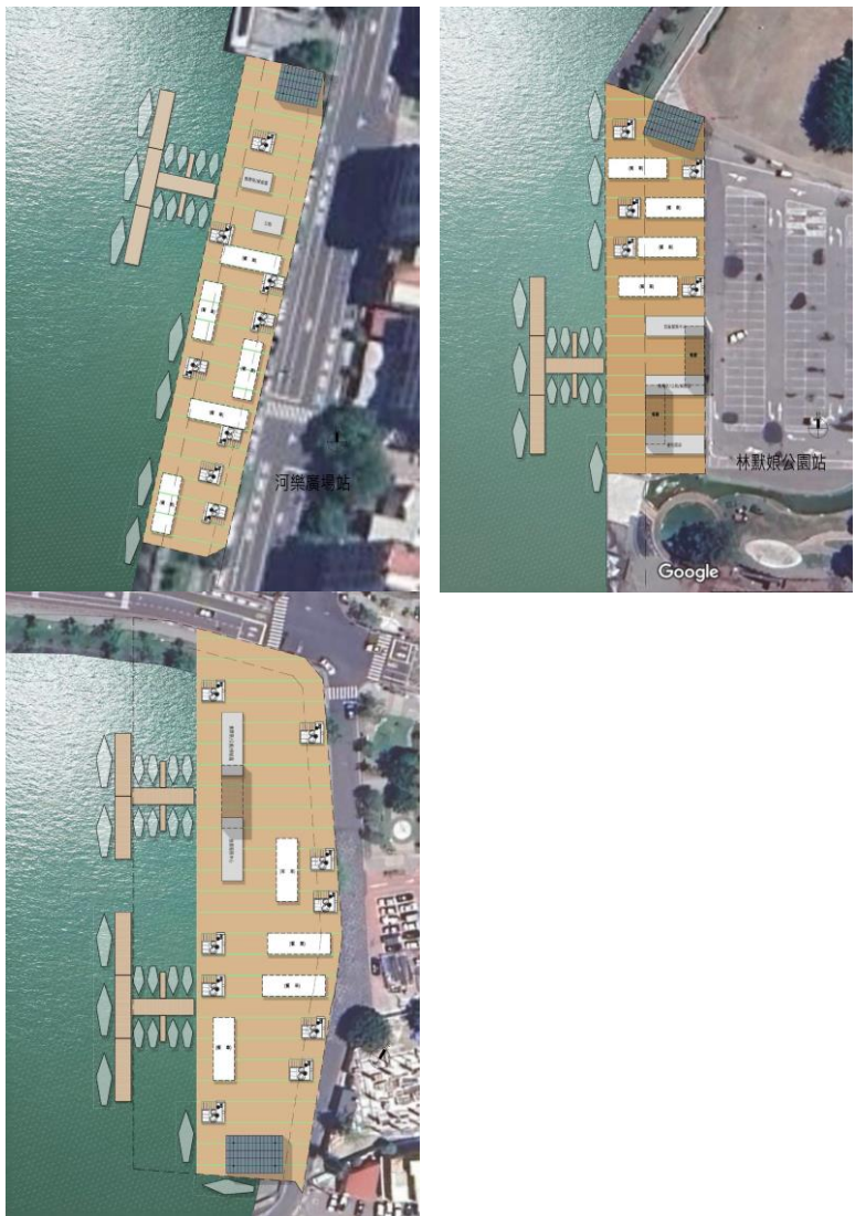
模擬示意圖
