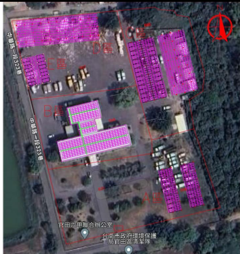
官田區清潔隊光電停車棚設置示意圖
